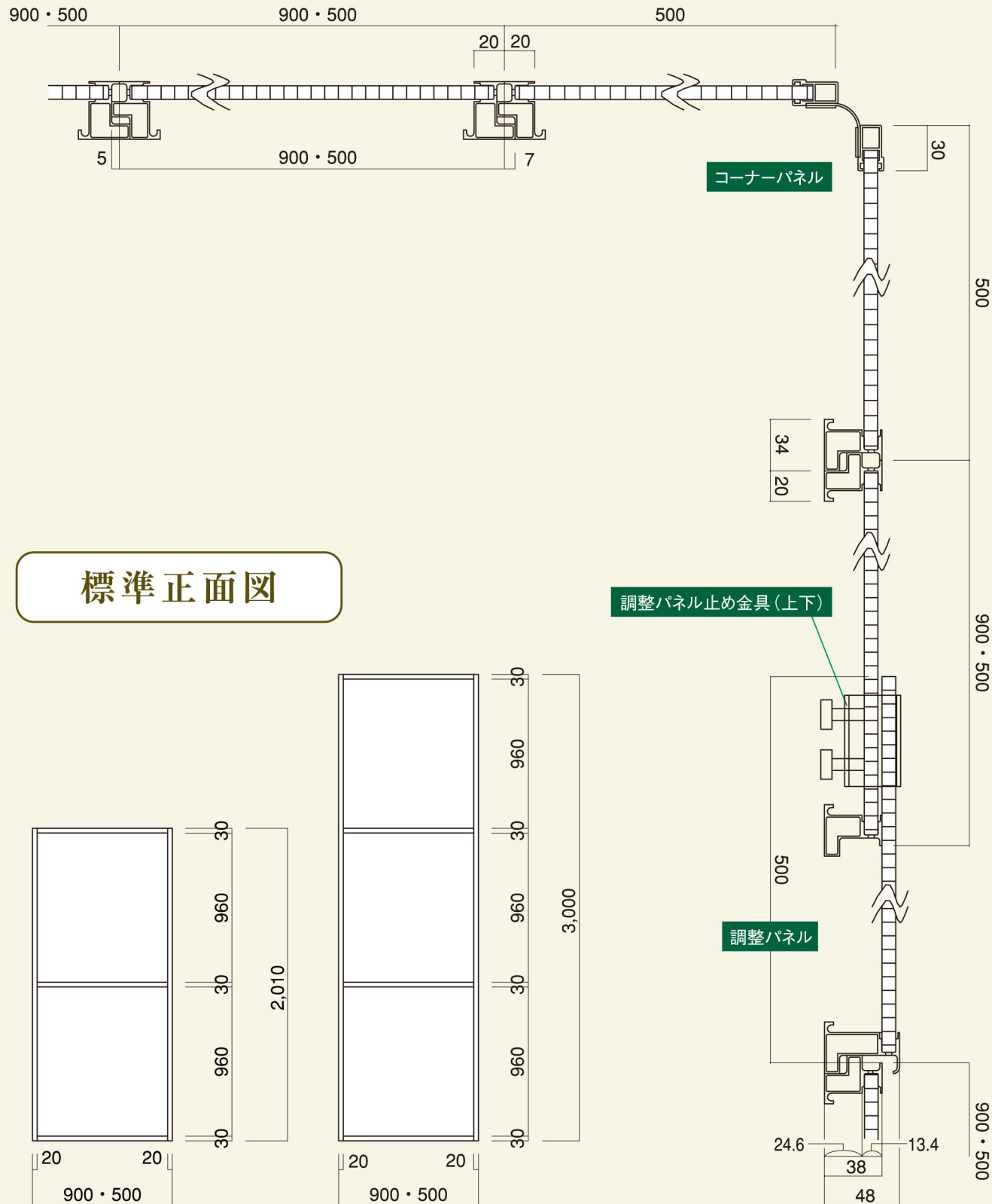
施工断面図
