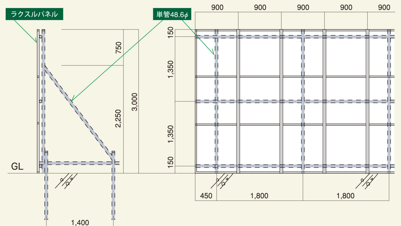
標準単管施行図
