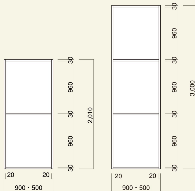
標準正面図
