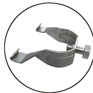
Vフック (一側足場用)
