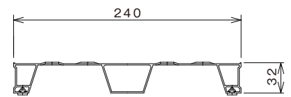
床材断面
