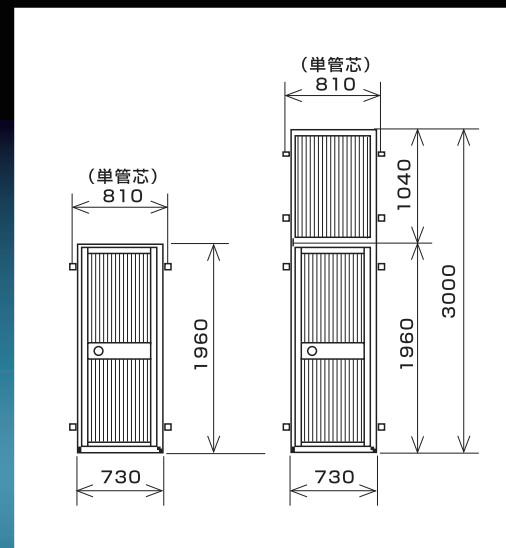
■ アルミくぐり戸
