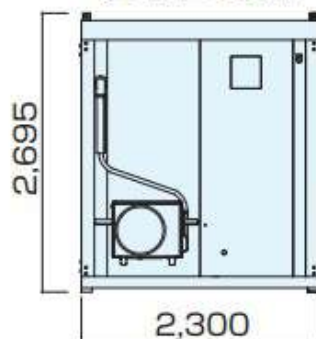
(立面図 妻側)
