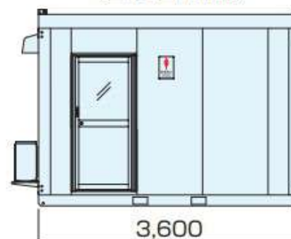
(立面図 桁側)
