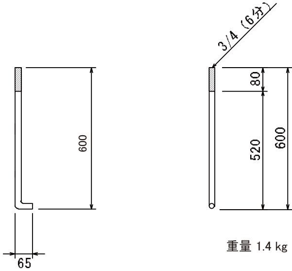
アンカーボルト
