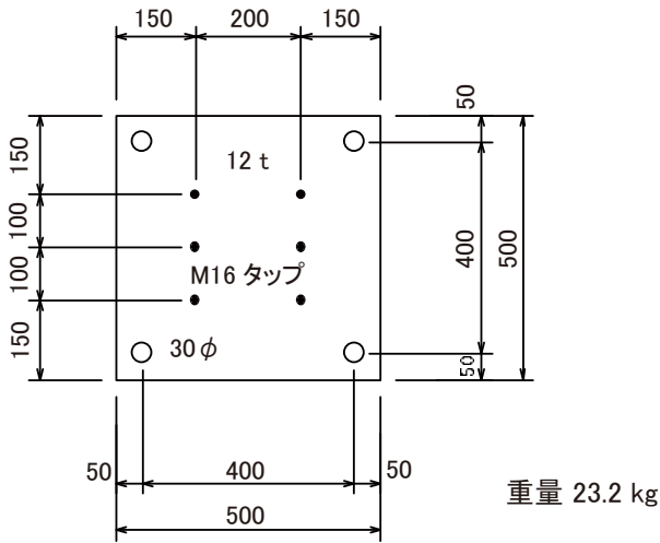
ベースプレート 12mm厚
